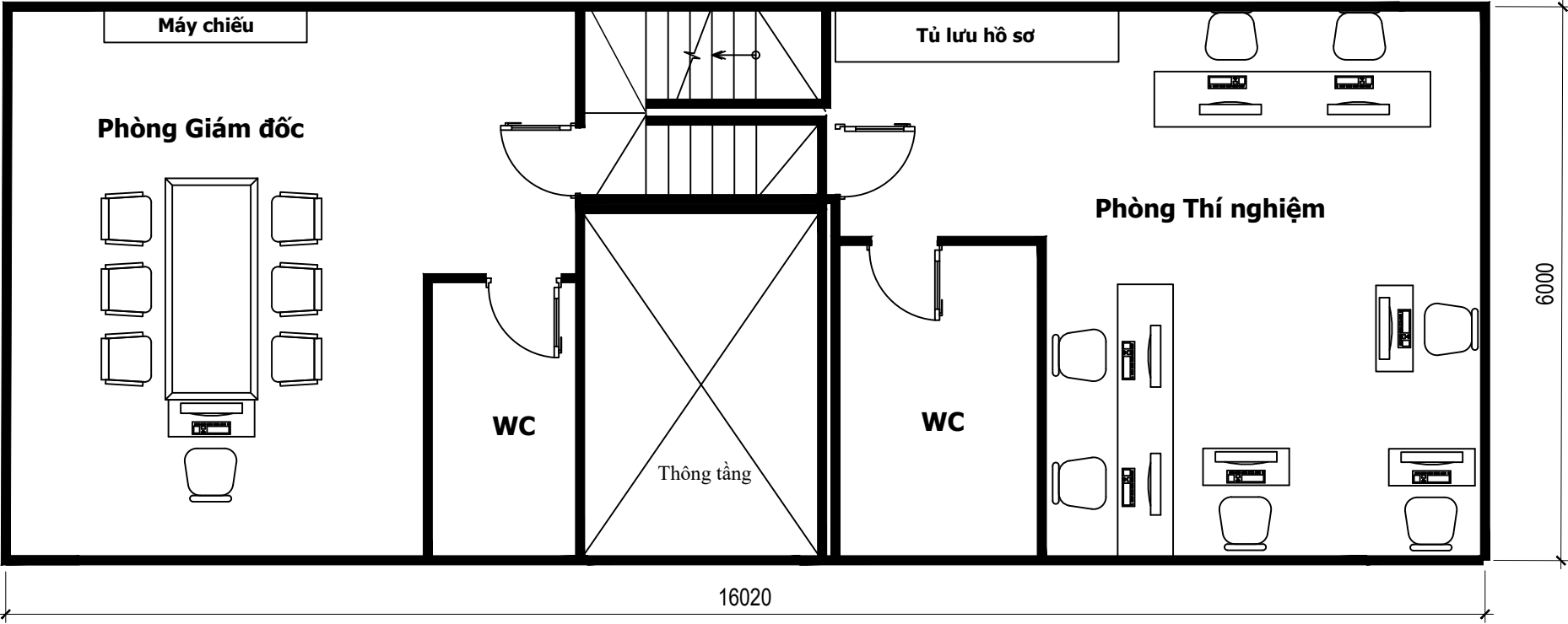
MẶT BẰNG LẦU 1
