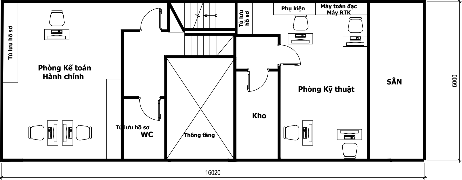
MẶT BẰNG LẦU 2
